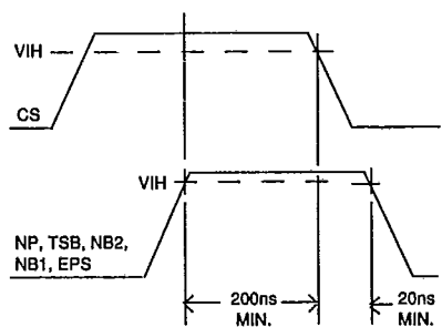
FIG. 11A CS
