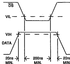
FIG. 10 DS
