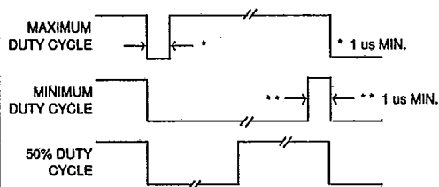
FIG. 5 ALLOWABLE TCP, RCP
